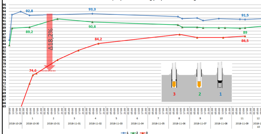
Jämförelse HMP36 i Vct0,32 (samma betong pall) olika monteringsätt
