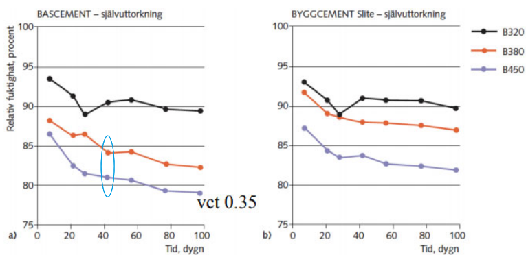
Figur 13. Exempel på uttorkningsförlopp vid självtorkning hos betong med a) Bascement och b) Byggcement Slite vid cementhalterna 320 kg/m 3 (vct = 0.55).
